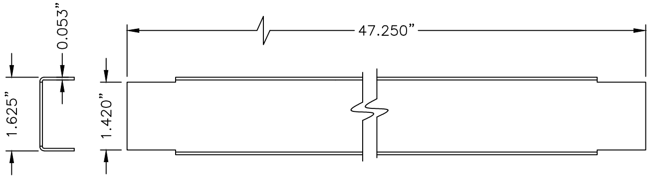
4 DOOR TOP & BOTTOM CLOSER 16GA. (.053) C.R.S.
